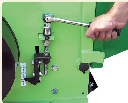
Facile millimetrica regolazione rullo. Easy millimetrical roller adjustment. Réglaçe millimétrique du rouleau arrière. Einfachste, millimeteregenaue. Höheneinstellung der Stützrolle.
